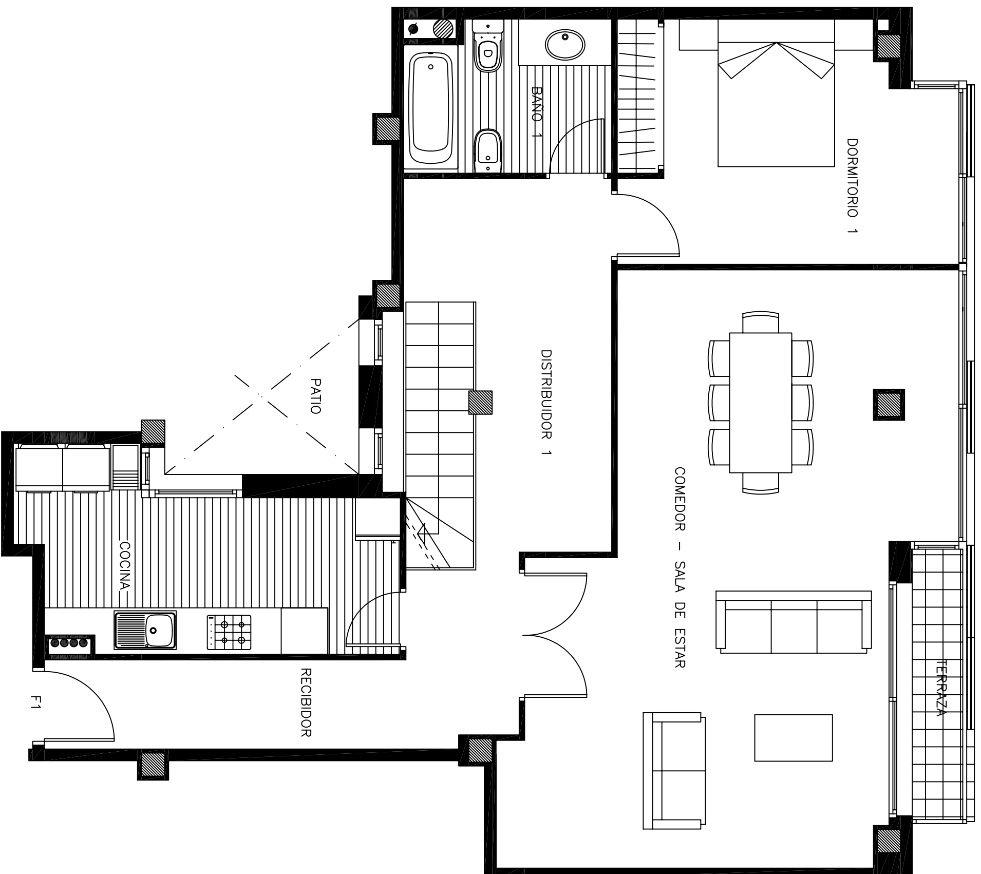
PLANTA PISOS 4 VIVIENDA TIPO F1 ESCALA GRAFICA
