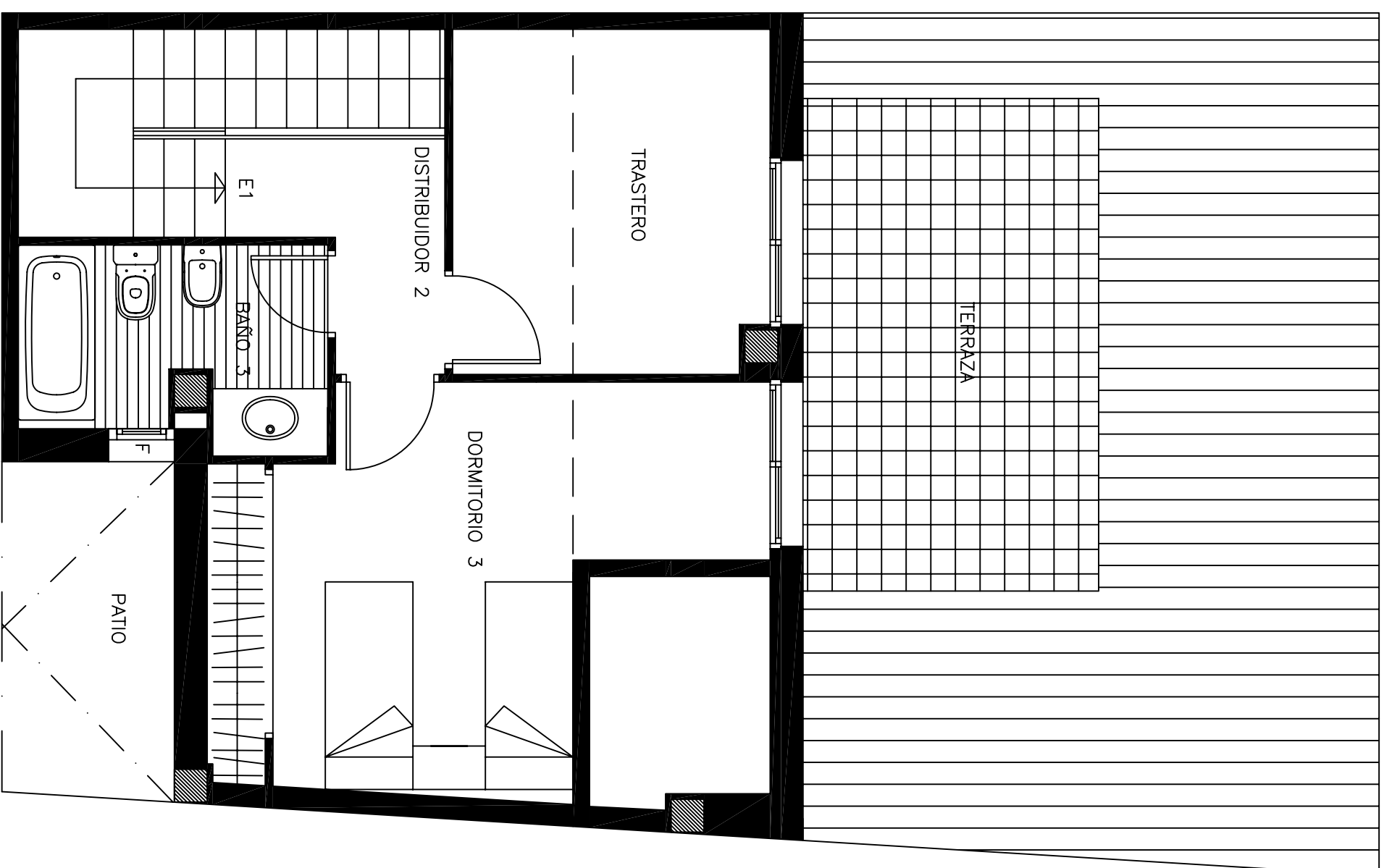
PLANTA PISOS BAJOCUBIERTA VIVIENDA TIPO E1 ESCALA GRAFICA
