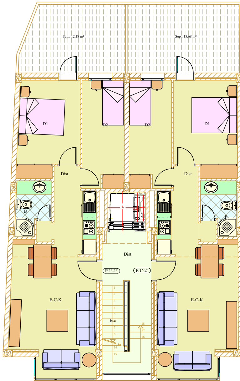
DISTRIBUCIÓN P.1ª
